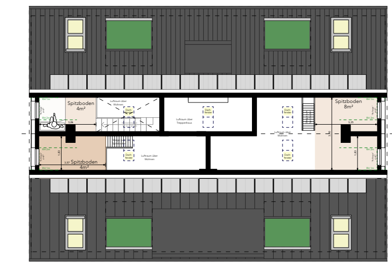
Spitzboden
