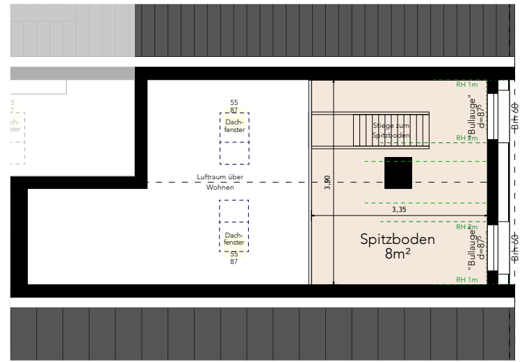
GRUNDRISS SPITZBODEN
